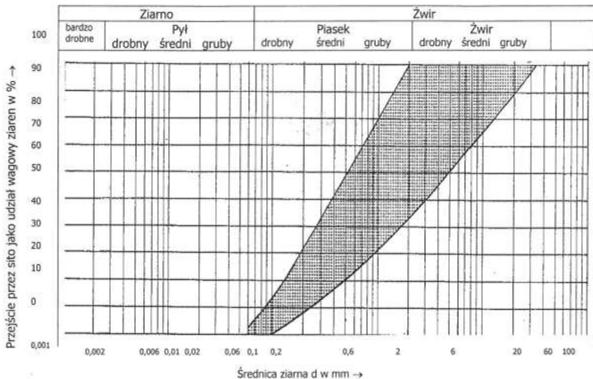
Rys. 2. Krzywa uziarnienia warstwy odsączającej
